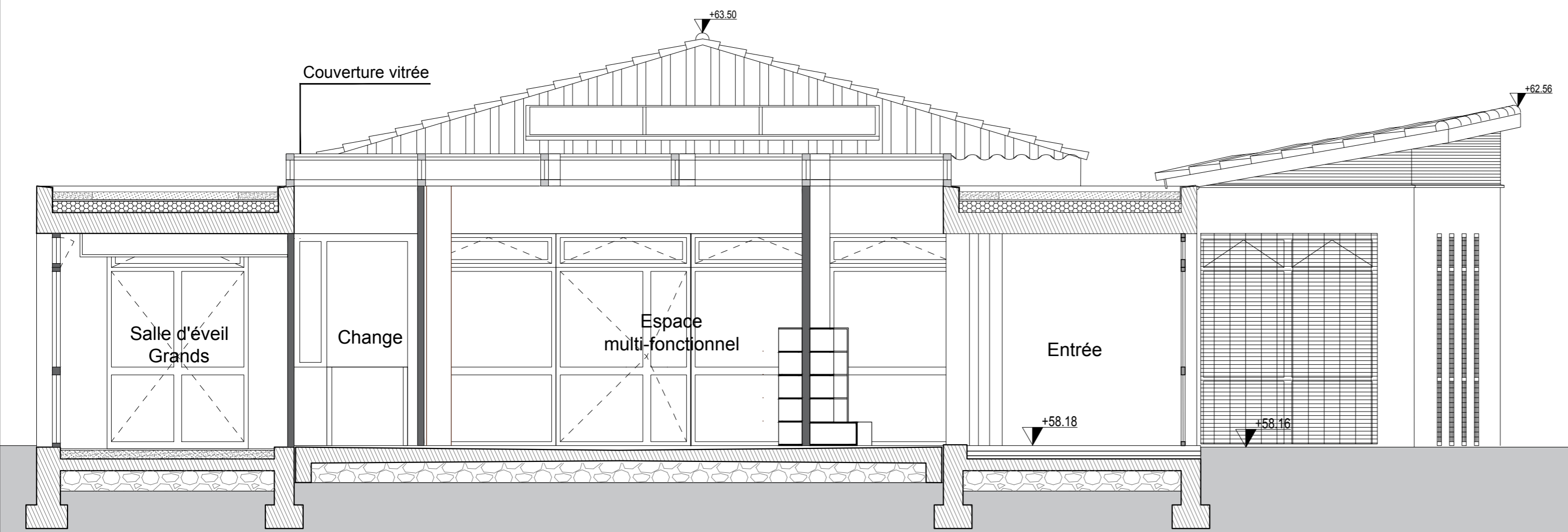
COUPE BB
