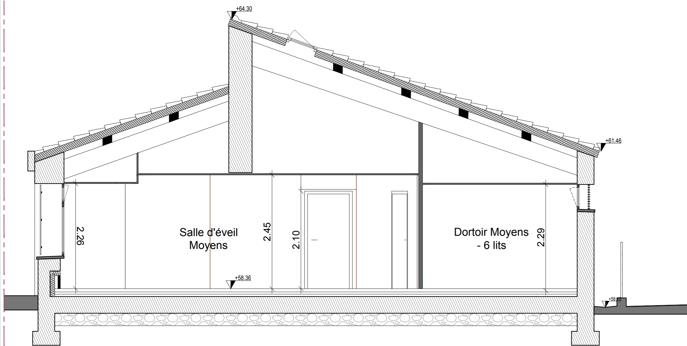
COUPE CC
